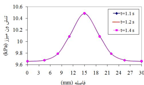
شکل (۴): نمودار تنش ون‌میزر برای سطح بالایی مدل بافت شامل غده در سه زمان متفاوت و در طول ۱ ثانیه دوم از زمان حل مسأله.
