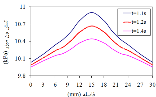
شکل (۵): نمودار تنش ون‌میزر برای سطح بالایی مدل بافت شامل شریان در سه زمان متفاوت و در طول ۱ ثانیه دوم از زمان حل مسأله.
