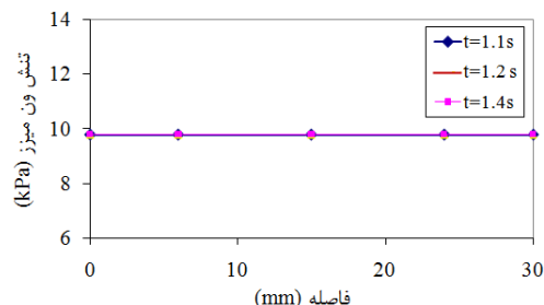
شکل (۳): نمودار تنش ون‌میزر بر روی سطح بالایی مدل بافت تنها و در ۳ زمان متفاوت در طول ۱ ثانیه دوم از زمان حل مسأله.
