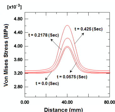
شکل (۶): نمودار تنش ون‌میزر بر روی سطح بالایی مدل بافت شامل شریان در چهار زمان متفاوت از مرحله سیستمولیک (۱۰).
